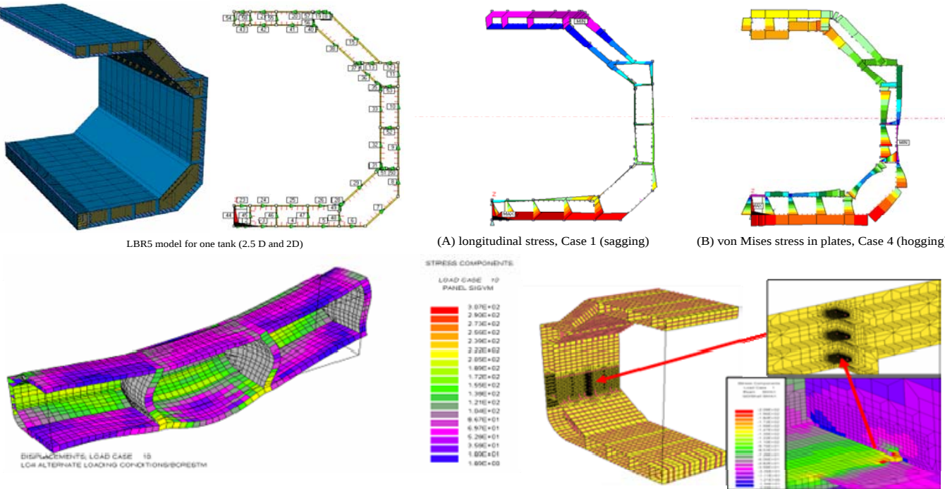
LNG Structural Optimisation
